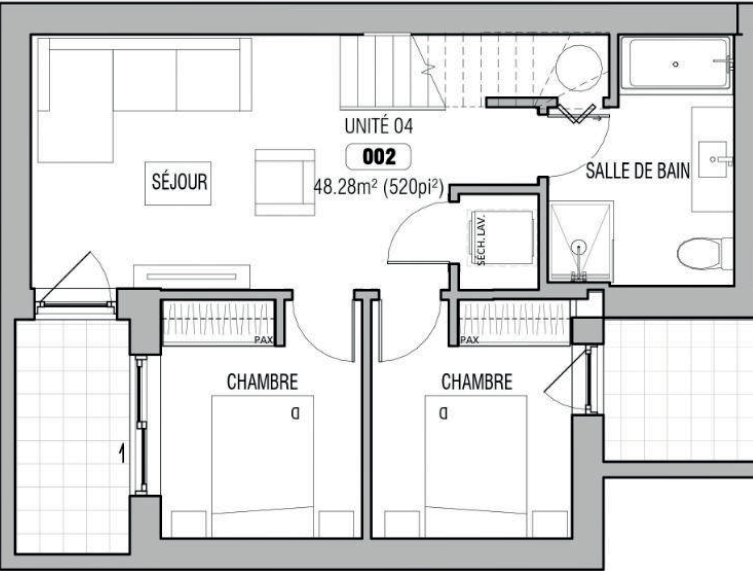
NIVEAU 1
